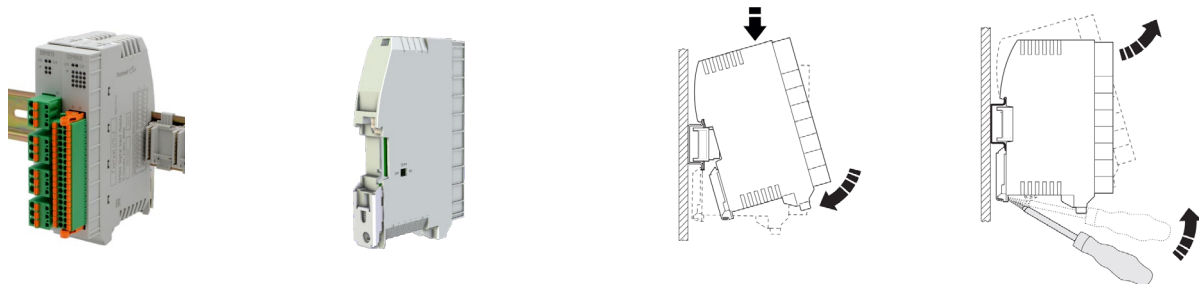
Габаритно-присоединительные размеры периферийных модулей
