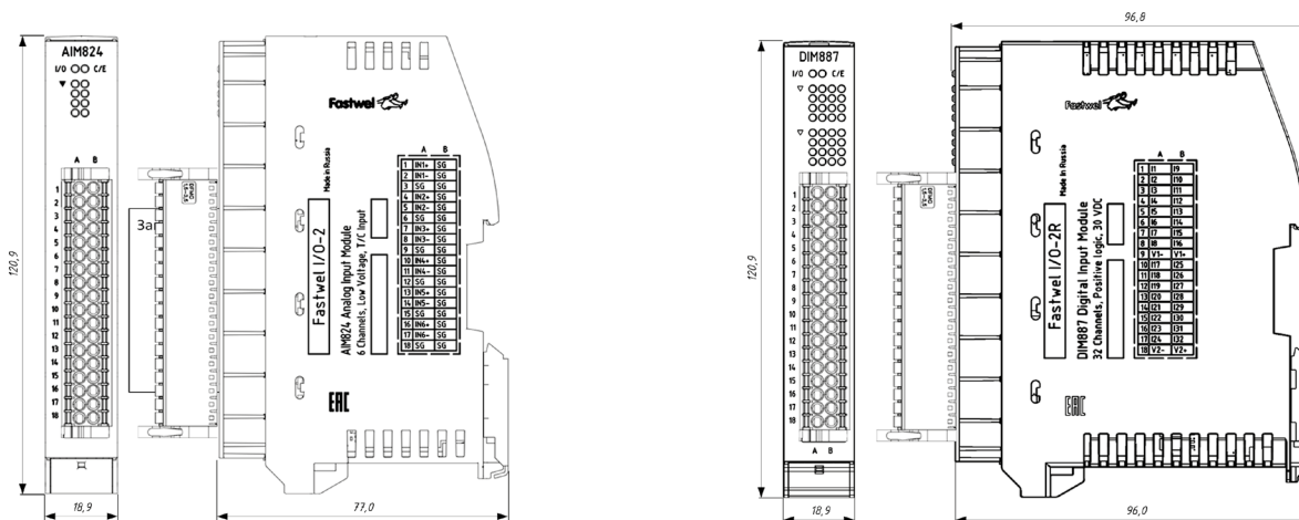
Габаритно-присоединительные размеры контроллеров
