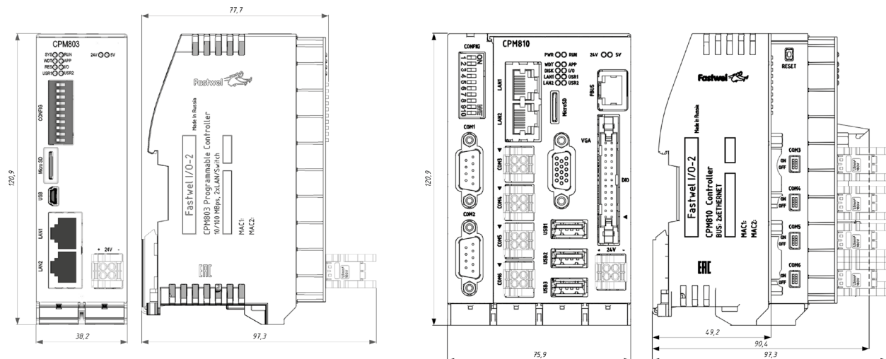
Габаритно-присоединительные размеры контроллеров
